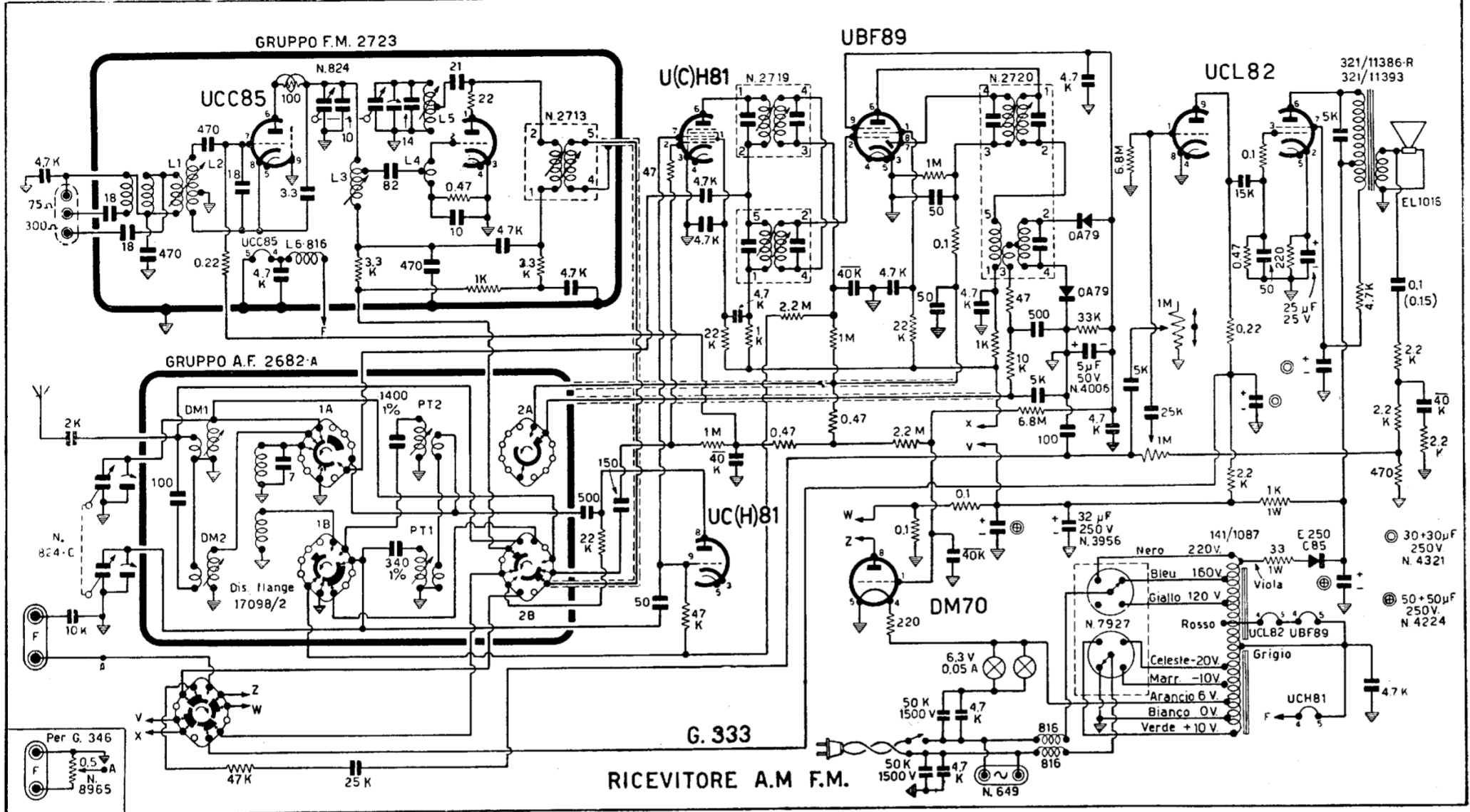
Schema elettrico del G.333-A
